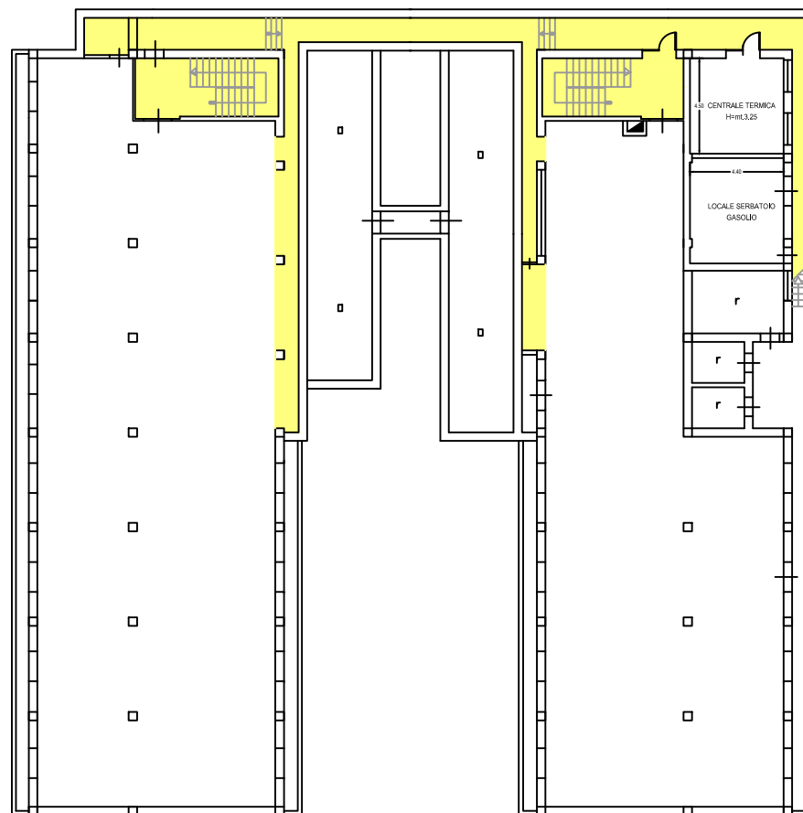
PIANTA PIANO INTERRATO
