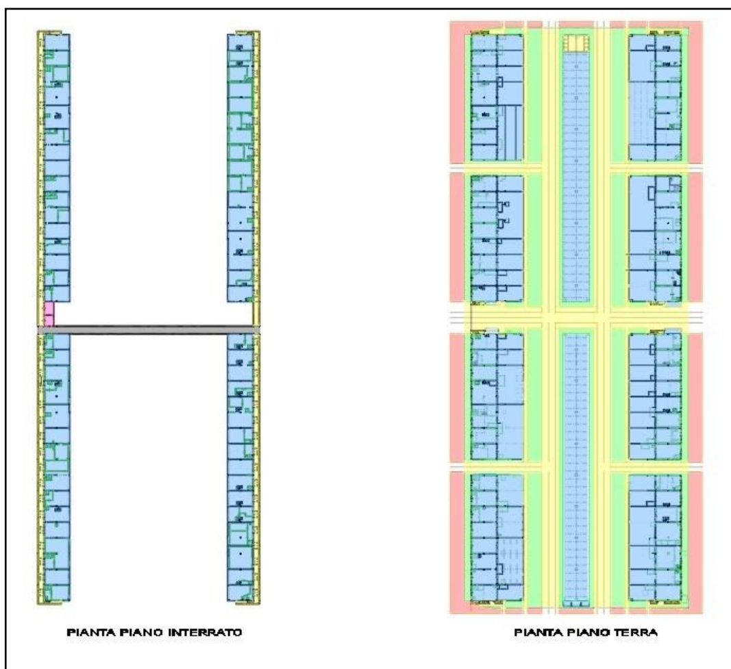
Fig. 4 – Planimetrie piano interrato e terra – piani tipo
